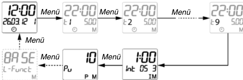
Abbildung 3: Navigationsstruktur Menü
